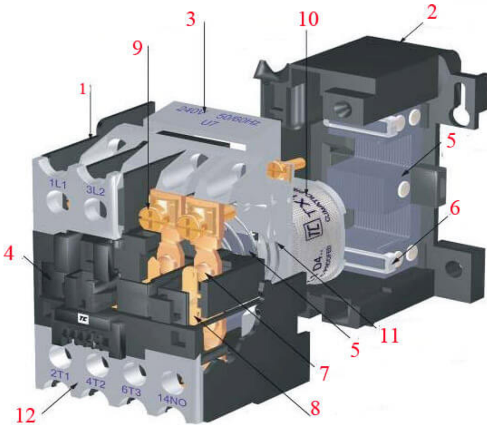
اجزای داخلی کنتاکتور
